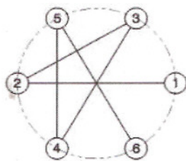
6 LUG BOLT PATTERN
